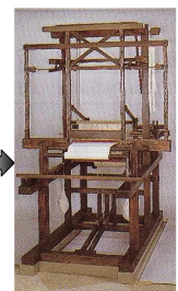
〔 国産 力織機〕 ( 機械 動力の段階)
